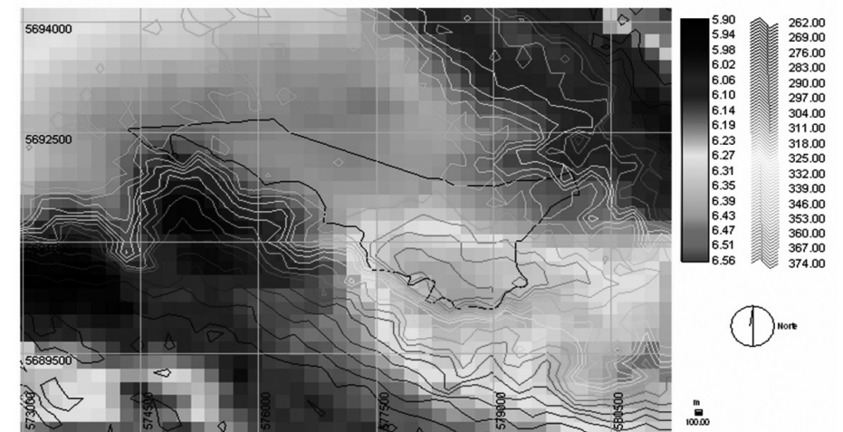
Figura 3: Viento transporte promedio ( m/s ) en la capa de mezcla considerando altura promedio ( H=693 m) del período analizado (año 2004), líneas: altura de la topografía (m) y área de expansión (línea sólida).
