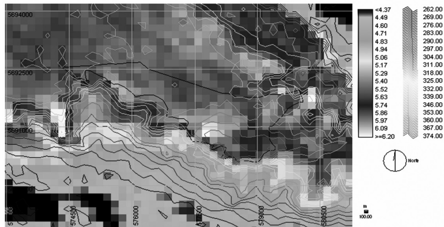
Figura 1: Viento transporte medio ( m/s ) en una capa de mezcla con altura mínima ( H=250 m) considerando datos del año 2004 (área planificada de expansión urbana, línea negra sólida)
