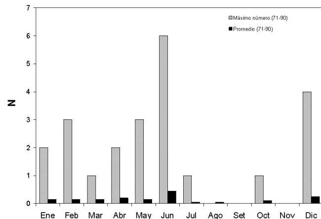
Figura 5: Número de días con tormenta de polvo en Neuquén Aero en el período 1971-1990.
