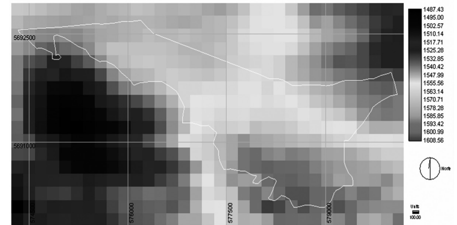
Figura 2: Índice de ventilación en el área de estudio ( m^2/s ) considerando una altura capa de mezcla mínima ( H=250 m) para casos en el año 2004 (área de expansión línea sólida blanca).
