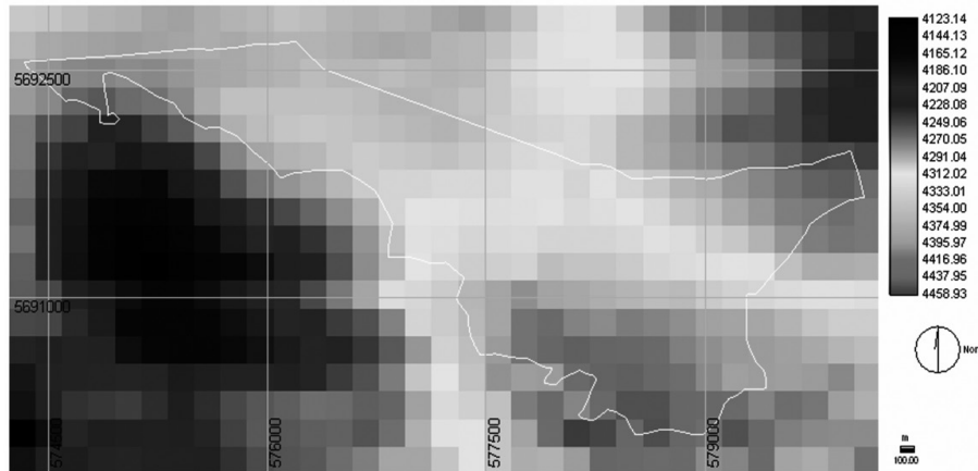
Figura 4: Índice de ventilación ( m^2/s ) considerando una capa de mezcla promedio de 693 m con información del año 2004 en el área de estudio (línea sólida blanca).
