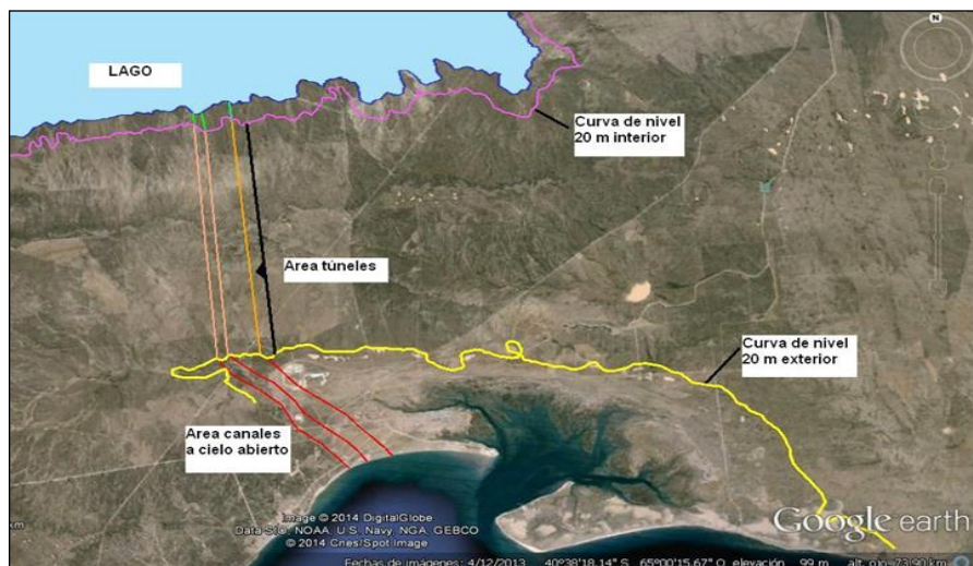
Figura 4. Propuesta de canales a cielo abierto y túneles. Imagen 3D Google Earth.
